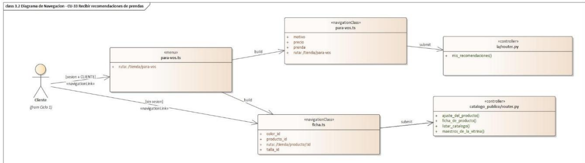
class 3.2 Diagrama de Navegación - CU-33 Recibir recomendaciones de prendas
