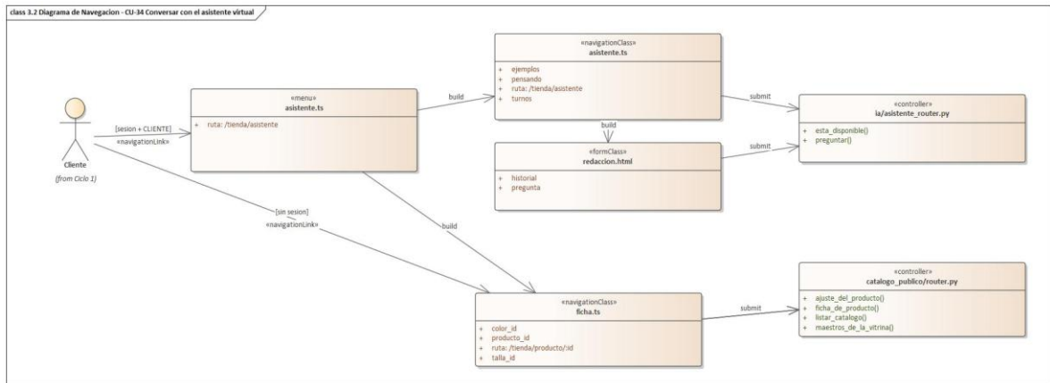
class 3.2 Diagrama de Navegación - CU-34 Conversar con el asistente virtual
