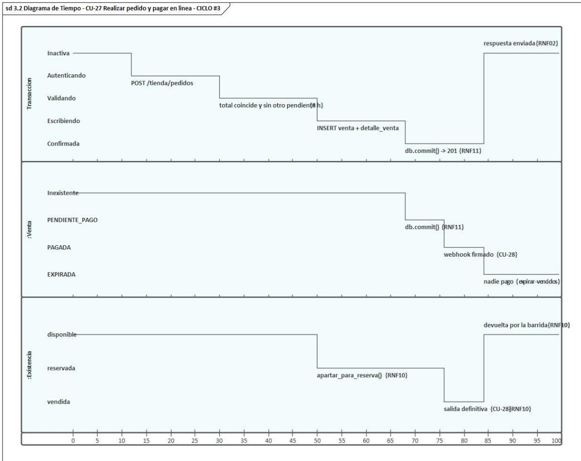
sd 3.2 Diagrama de Tiempo - CU-27 Realizar pedido y pagar en línea - CICLO #3
