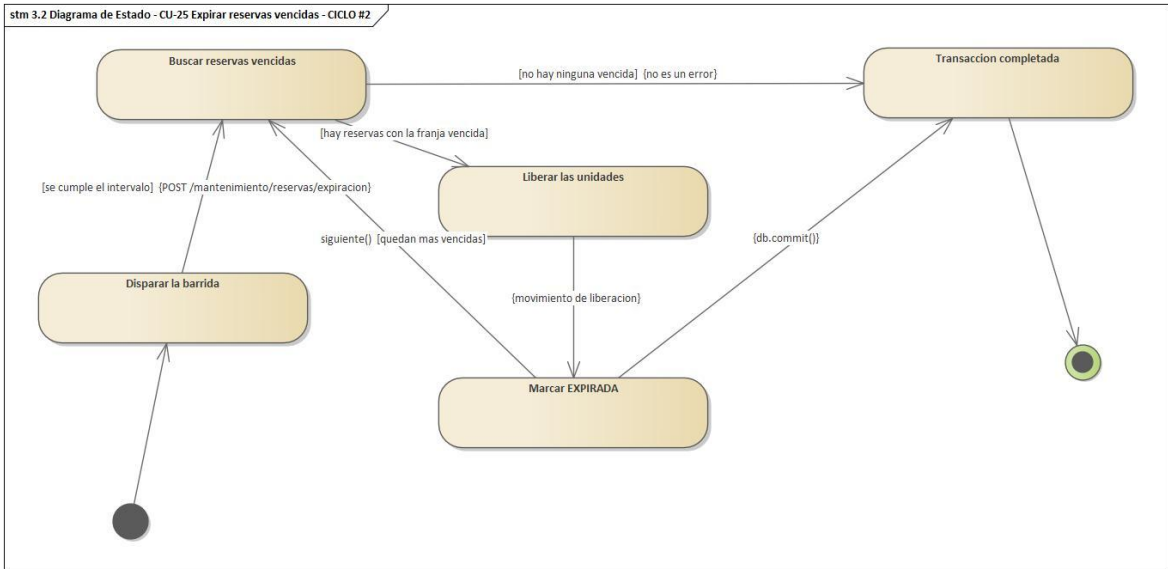
stm 3.2 Diagrama de Estado - CU-25 Expirar reservas vencidas - CICLO #2
