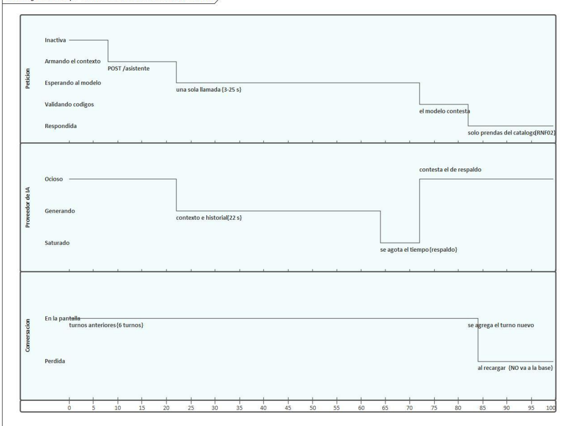
sd 3.2 Diagrama de Tiempo - CU-34 Conversar con el asistente virtual - CICLO #3
