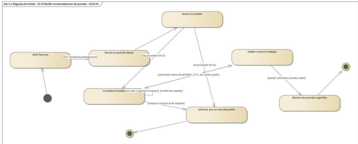
stm 3.2 Diagrama de Estado - CU-33 Recibir recomendaciones de prendas - CICLO #3
