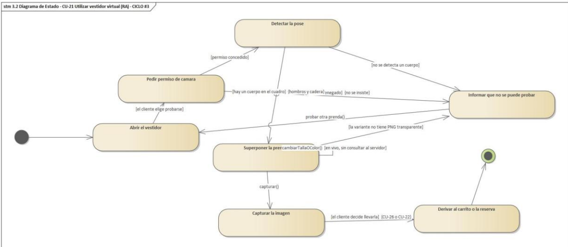
stm 3.2 Diagrama de Estado - CU-21 Utilizar vestidor virtual (RA) - CICLO #3
