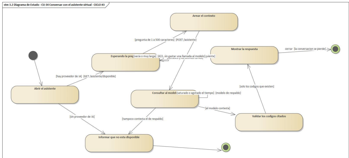
stm 3.2 Diagrama de Estado - CU-34 Conversar con el asistente virtual - CICLO #3
