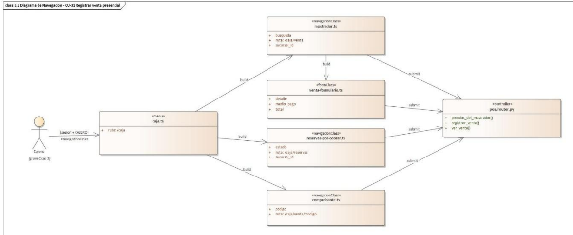
class 3.2 Diagrama de Navegación - CU-31 Registrar venta presencial
