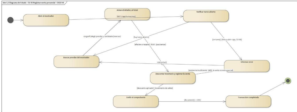
stm 3.2 Diagrama de Estado - CU-31 Registrar venta presencial - CICLO #3
